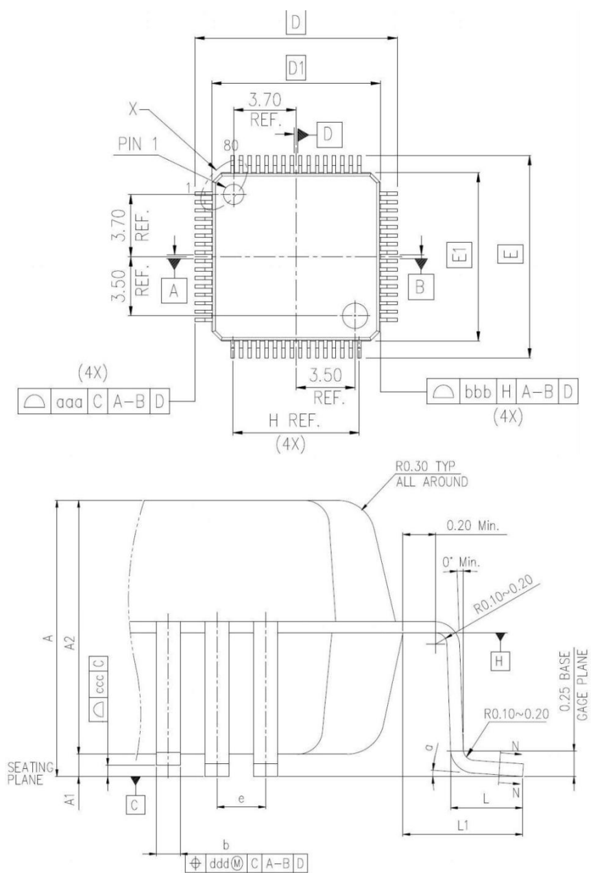
封装图
