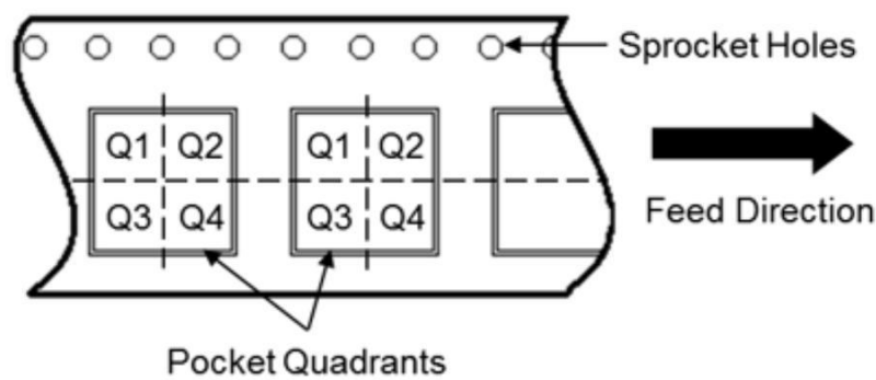
Reel Dimensions
