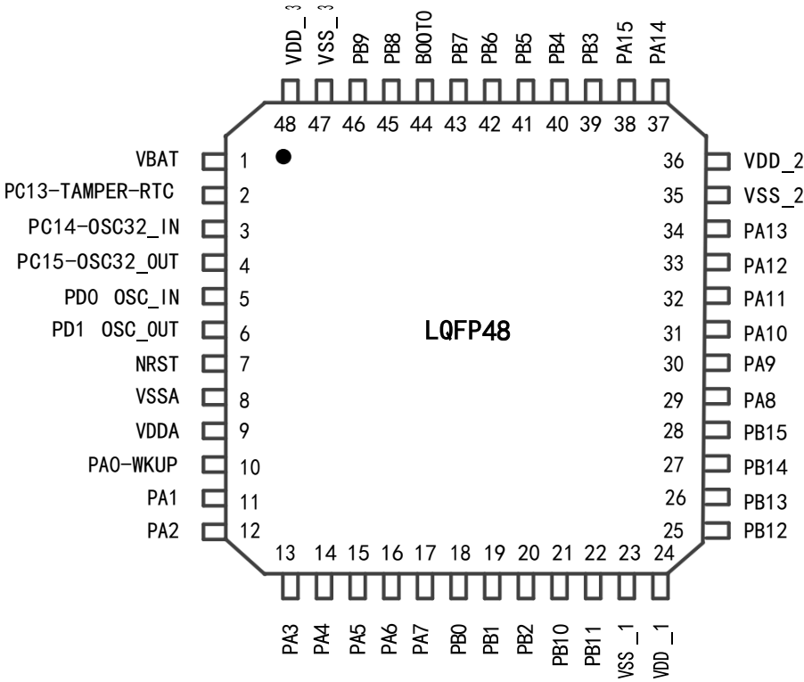
引脚分布图
