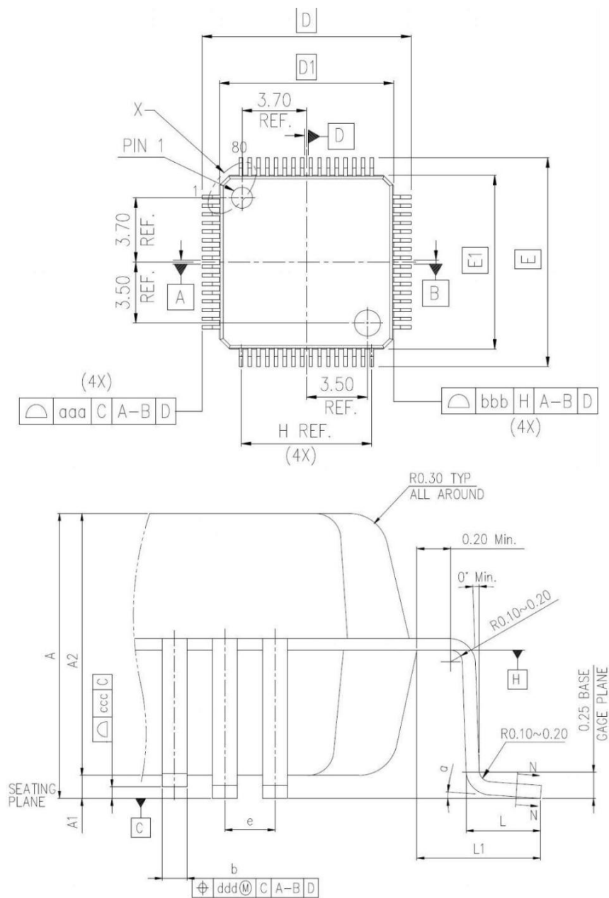
封装图
