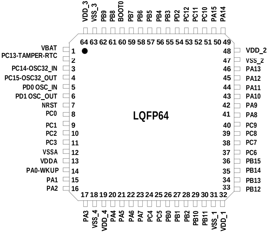
引脚分布图
