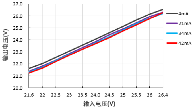
输出电压Vs输入电压@B2424S-1WR2
