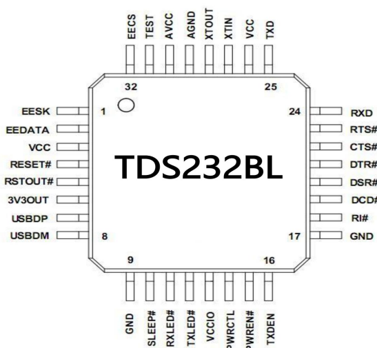
图一 引脚图 QFP32 封装
