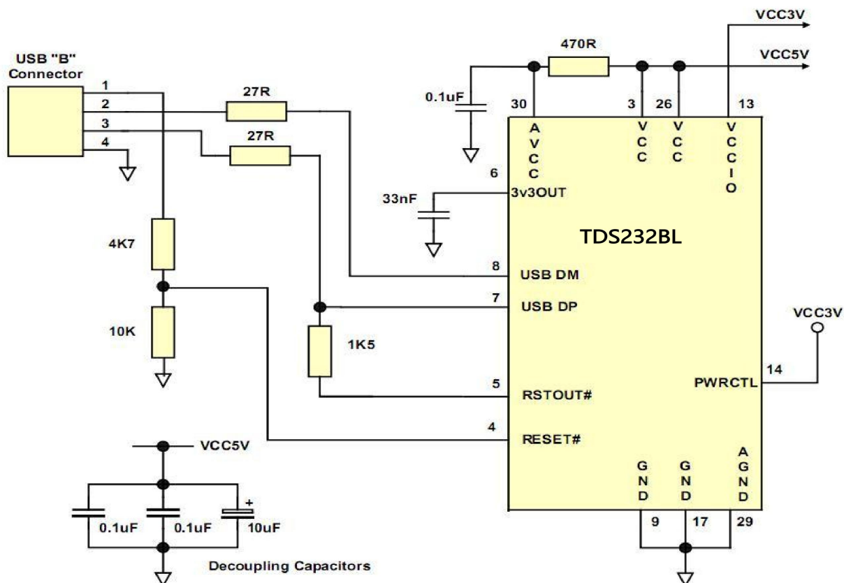
图 15 具有 3.3V 逻辑驱动/电源电压的自供电电路
