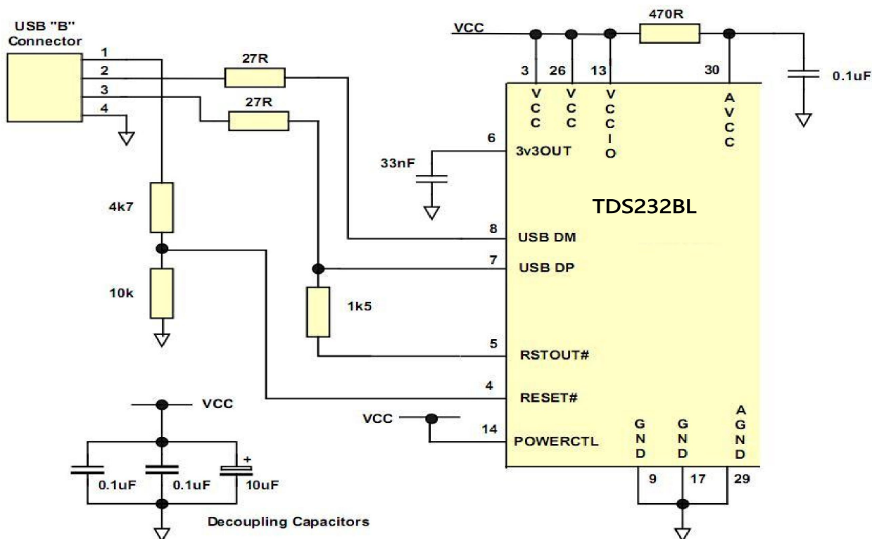
图 8 USB 自供电配置
