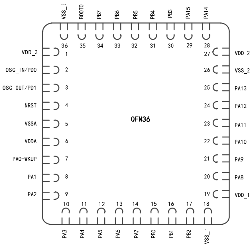
引脚分布图
