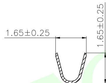
SEC: A-A
