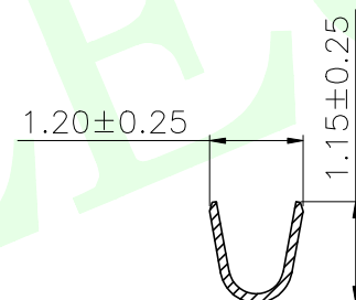
SEC: B-B
