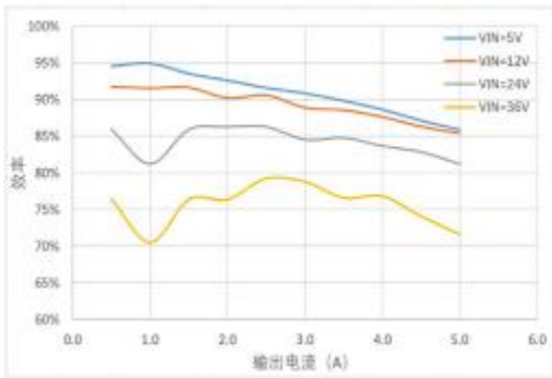
输出电流 vs 效率 ( V_{OUT}=3.3V )
