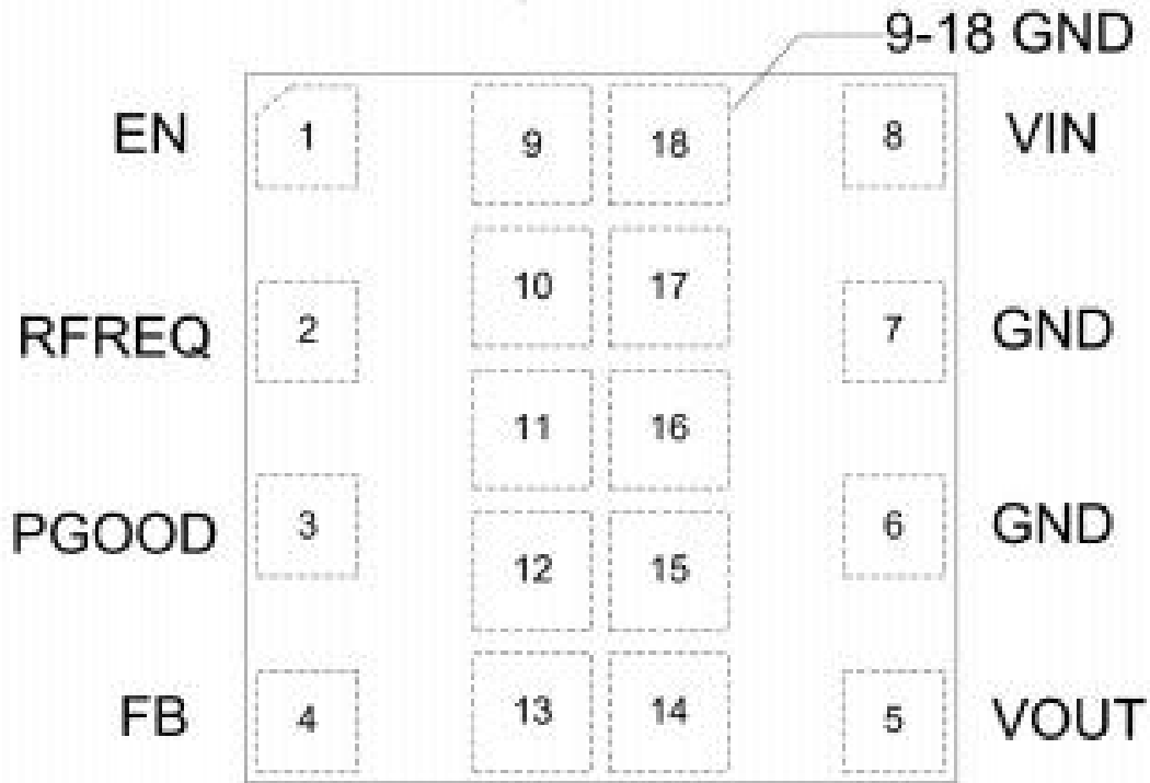
顶视图 (透视)
