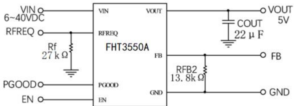
5V 输出典型应用电路
