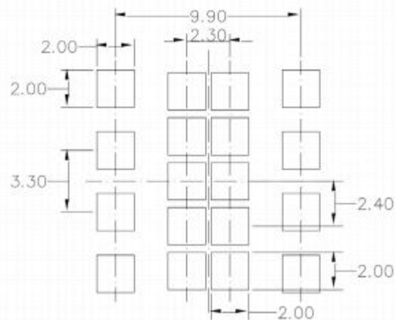
推荐焊盘
