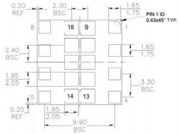
底视图
