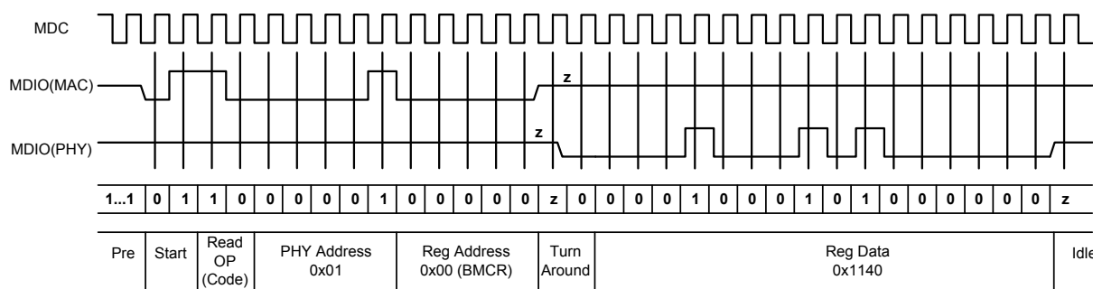
图6.读取周期
