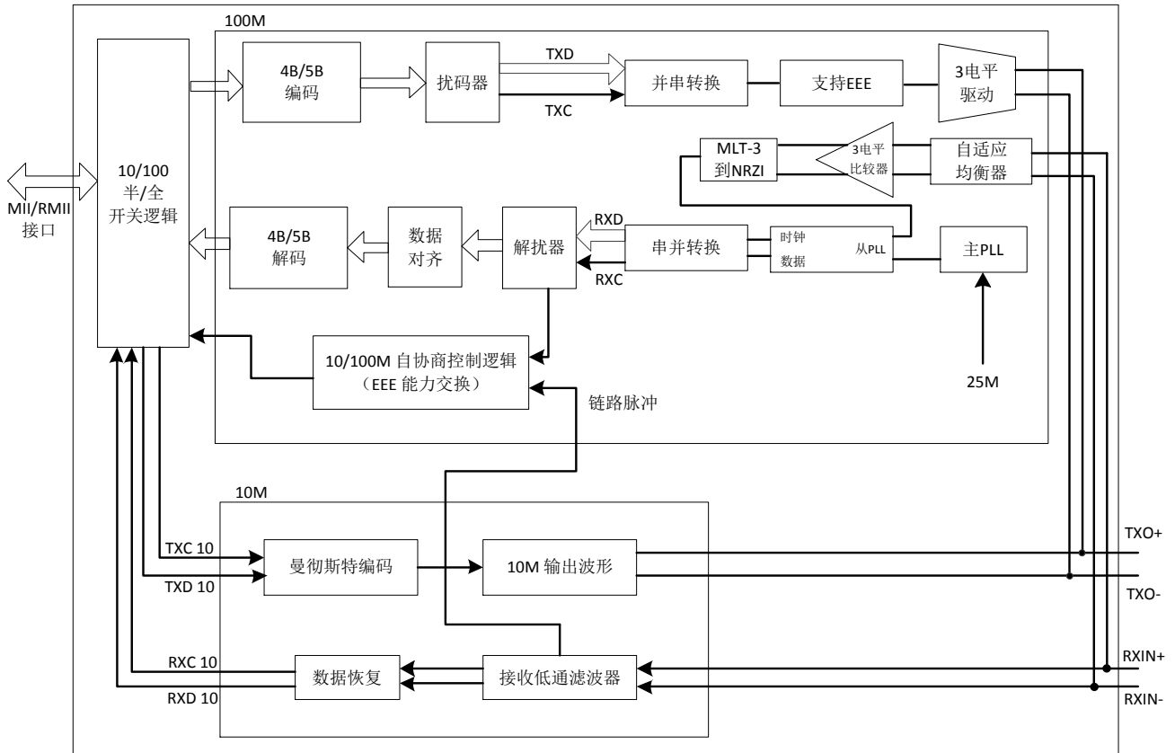
图 1. 内部框图
