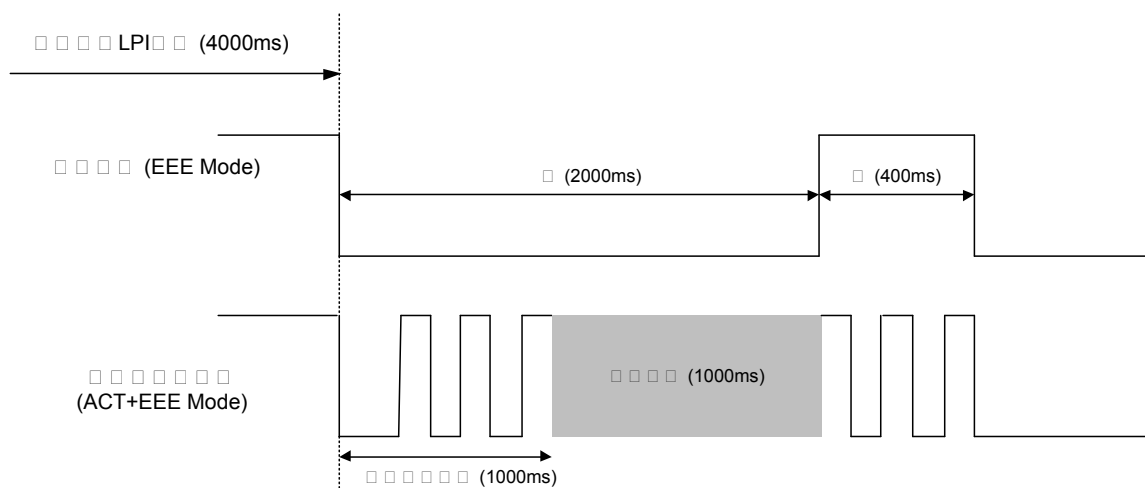
图 14.EEE LED 行为
