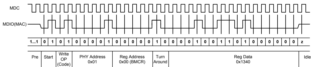
图7.写入周期
