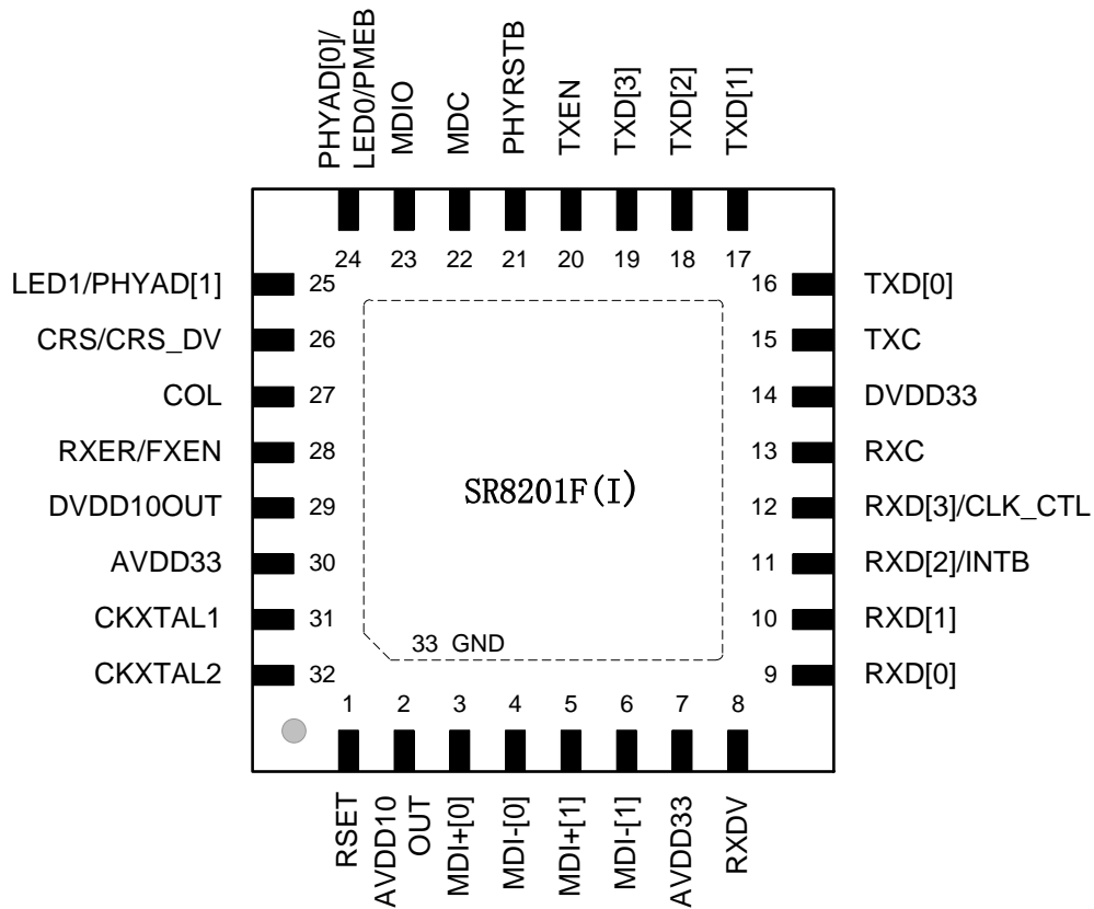
图 3. SR8201F(I) QFN-32封装图
