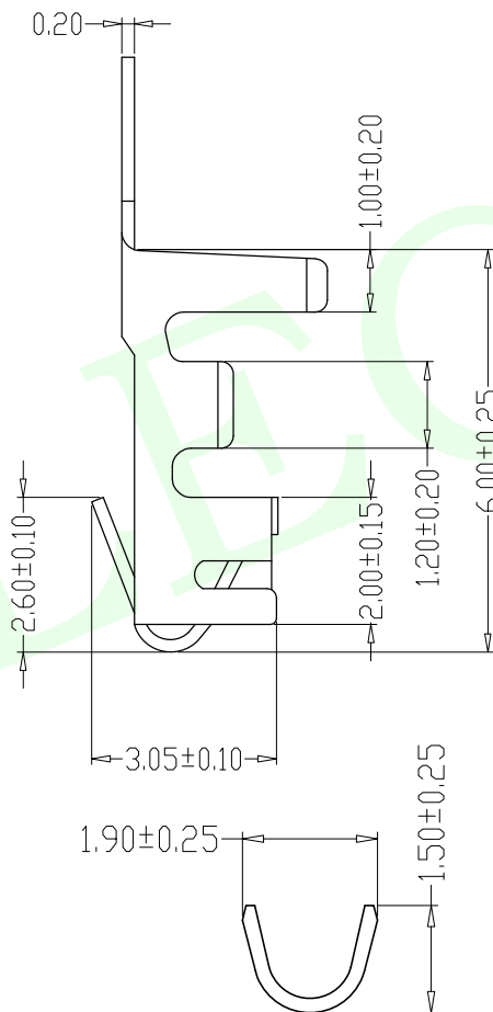
SEC: B-B
