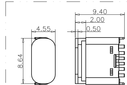
加塞子示意图 SCALE 2:1
