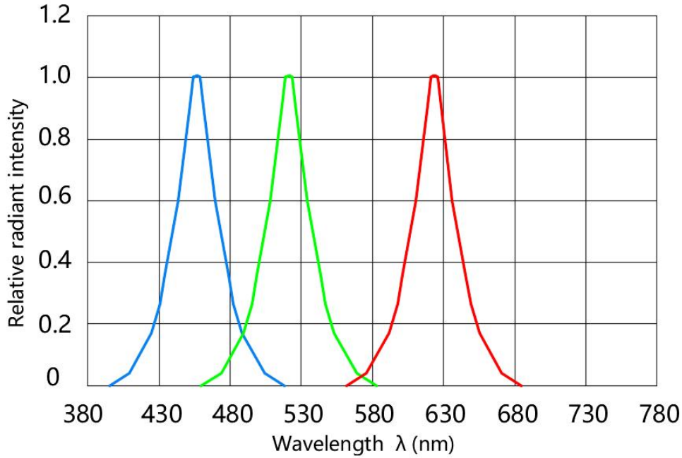
光谱分布曲线 Relative Spectral Distribution
