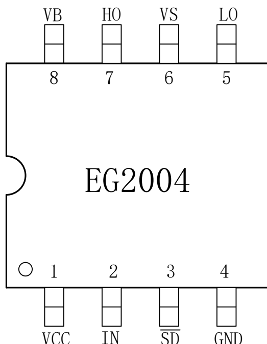
图 4-1. EG2004 管脚定义
