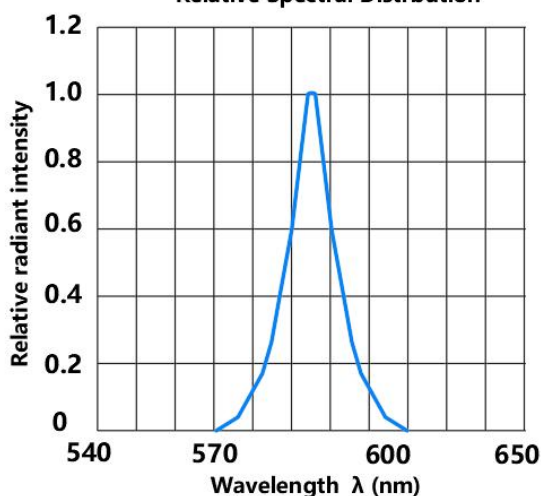
光谱分布曲线 Relative Spectral Distribution
