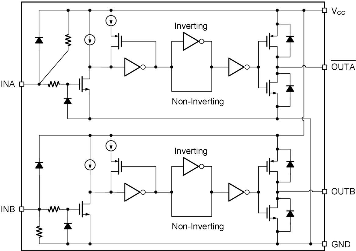
IX4428NTR-MS 功能框图
