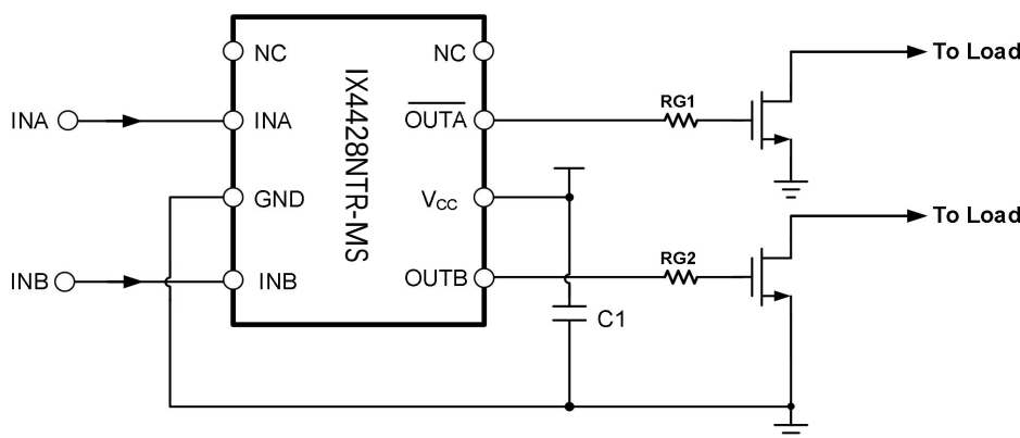
IX4428NTR-MS 典型应用电路图
