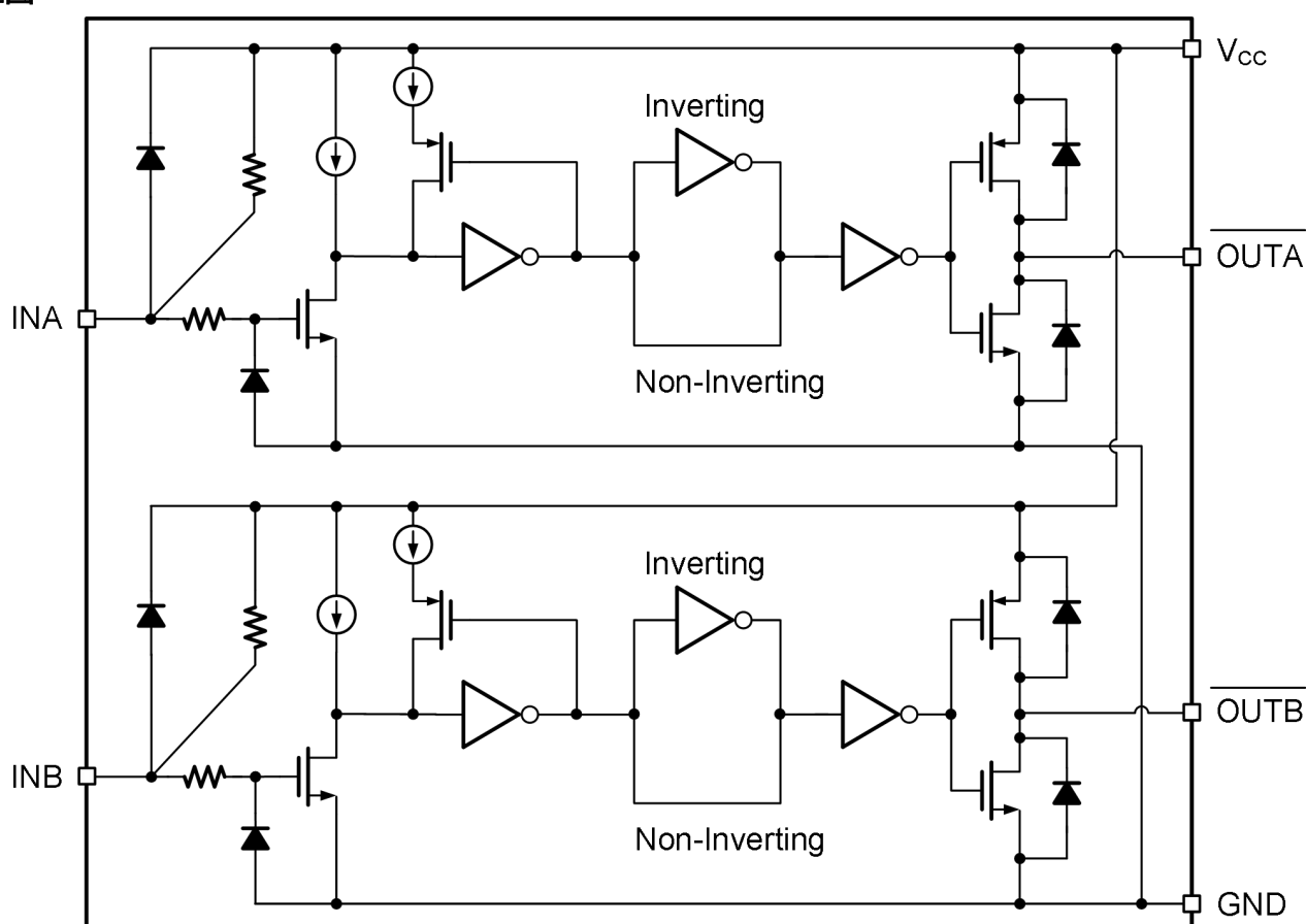
IX4426NTR-MS 功能框图
