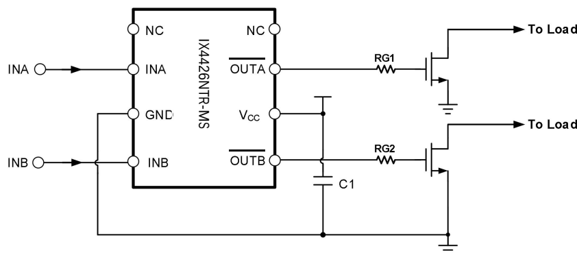
IX4426NTR-MS 反相典型应用电路图
