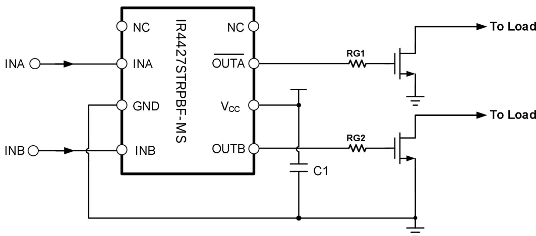
IR4427STRPBF-MS典型应用电路图
