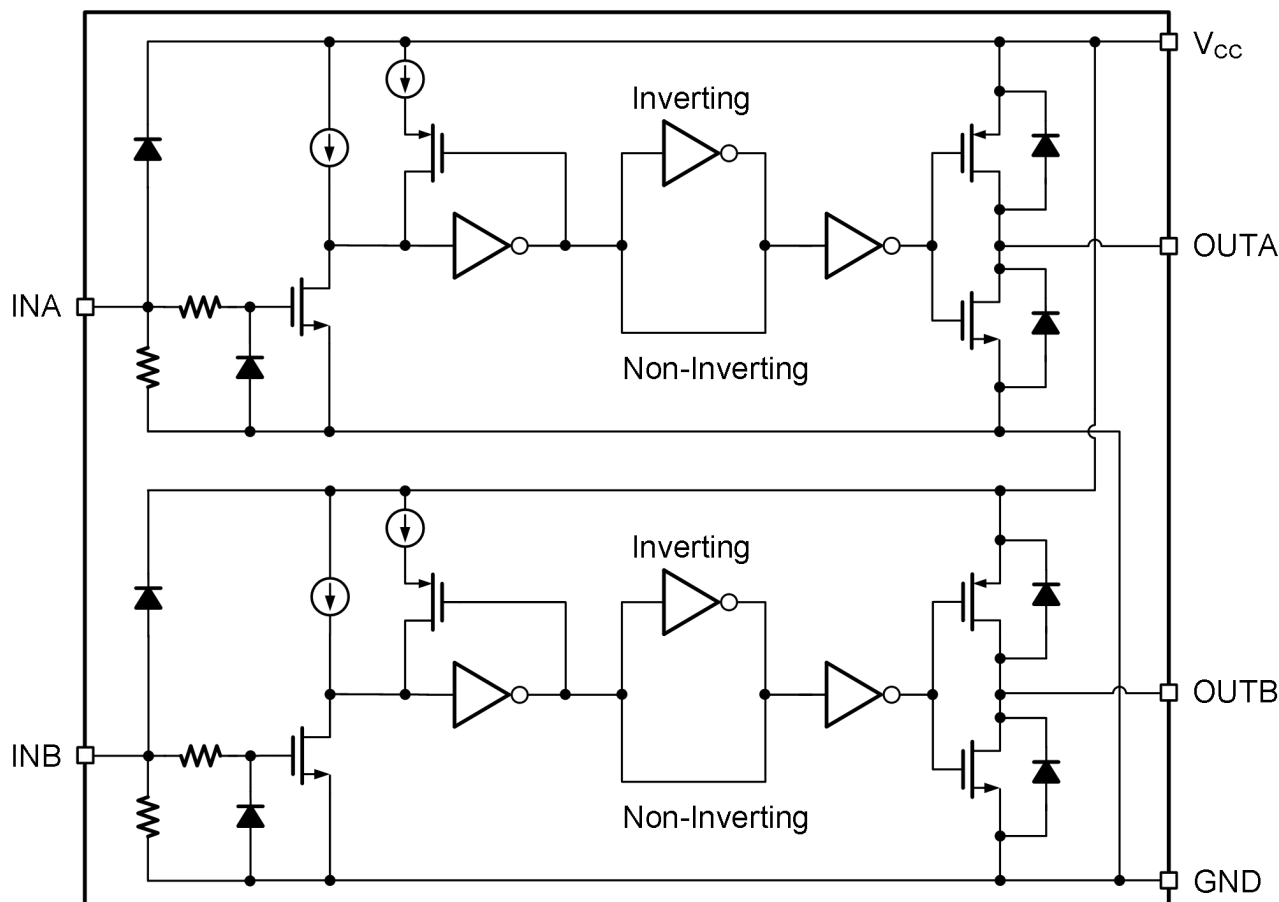
IR4427STRPBF-MS 功能框图
