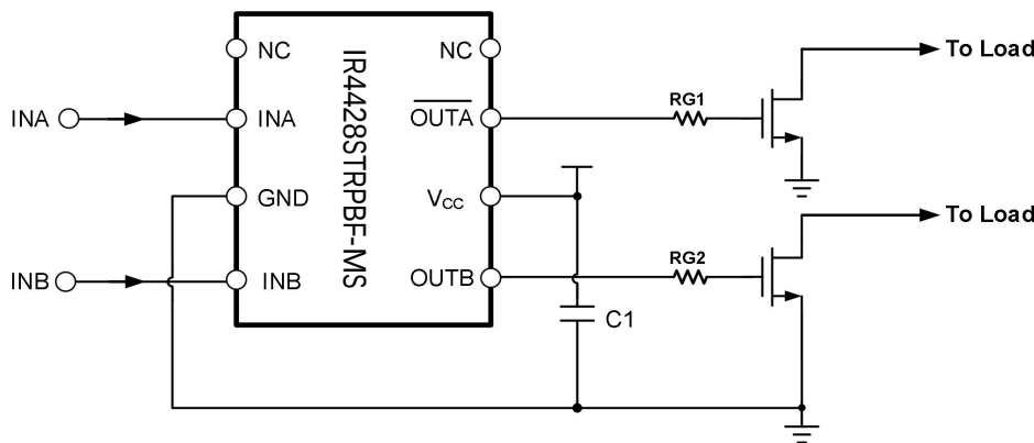
IR4428STRPBF-MS 典型应用电路图
