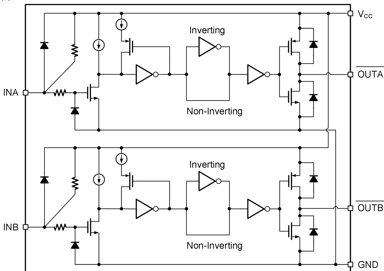
IR4426STR-MS功能框图
