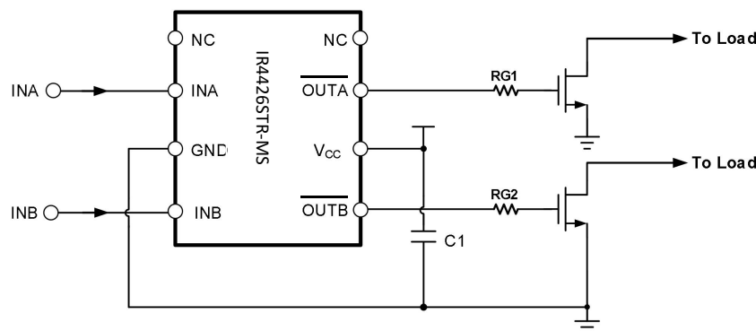
IR4426STR-MS反相典型应用电路图
