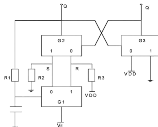
图 4 74HC4053A 实现的防抖动电路
