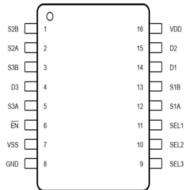
DIP-16/SOP-16/QSP-16/TSSOP-16
