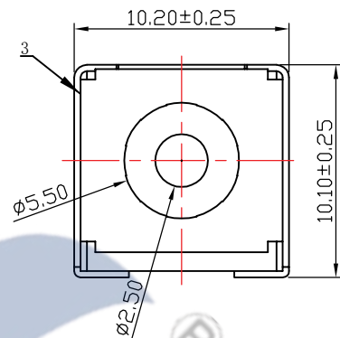
φ5.50mm公头详图
