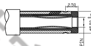
φ5.50mm公头详图
