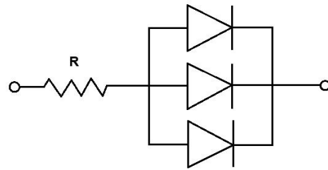
电路模式 B Circuit model B
