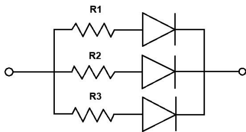
电路模式 A Circuit model A
