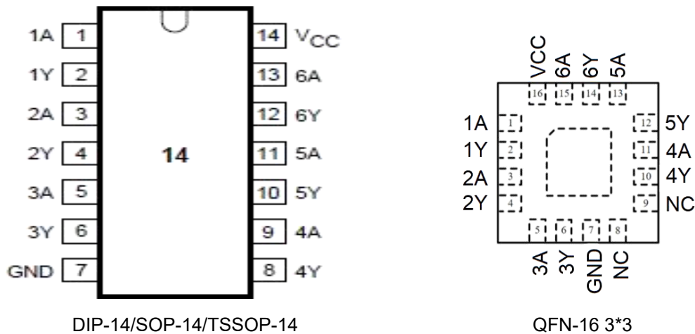
图 3、引脚排列图
