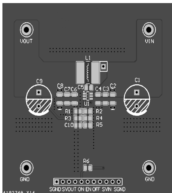
Top Layer
