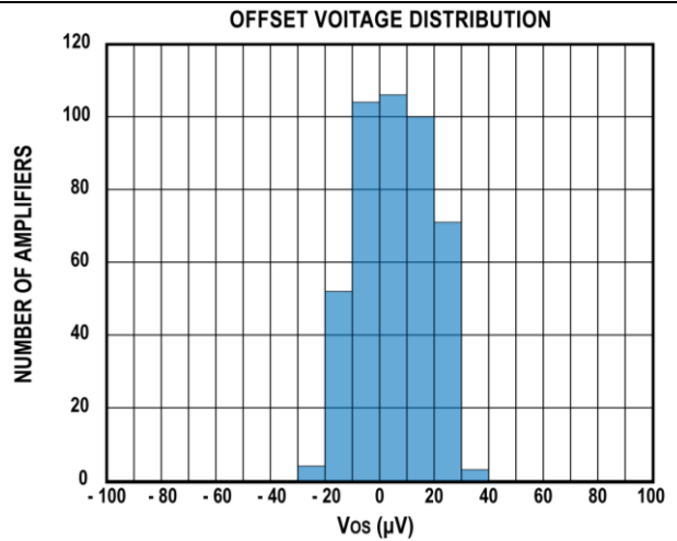
图4. 125 °C 失调电压分布, SOIC-8 封装
