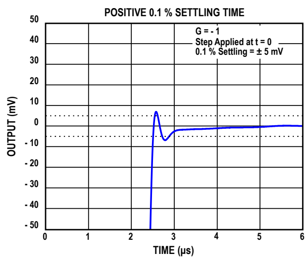
图23. 0.1 % 正建立时间
