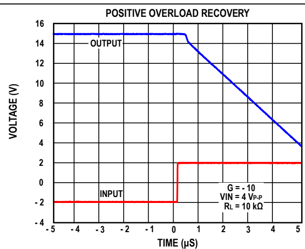
图18. 负过载恢复
