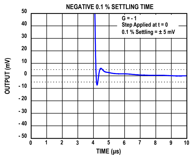
图24. 0.1 % 负建立时间
