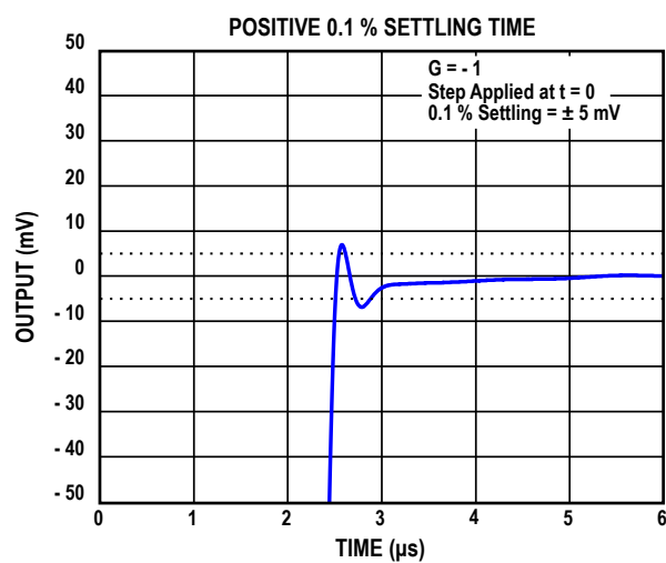
图23. 0.1 % 正建立时间
