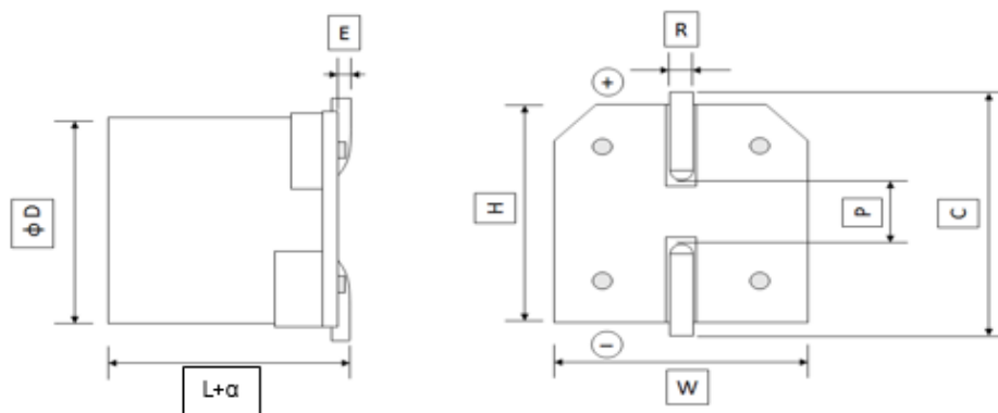
Fig. 2 Dimension
