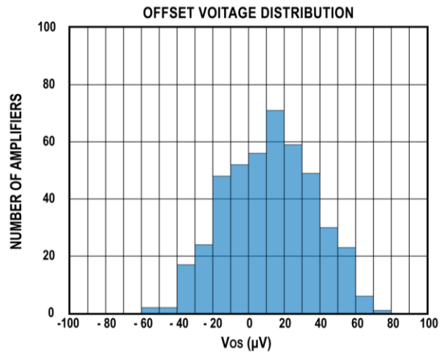
图2. -40 °C 失调电压分布，SOIC-8 封装
