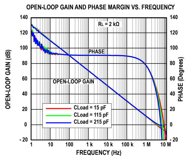
图12. 开环增益和相位与频率的关系
