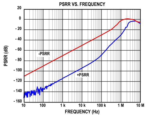
图20. 电源抑制比与频率的关系
