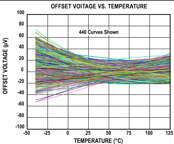
图5. 失调电压与温度的关系，SOIC-8 封装
