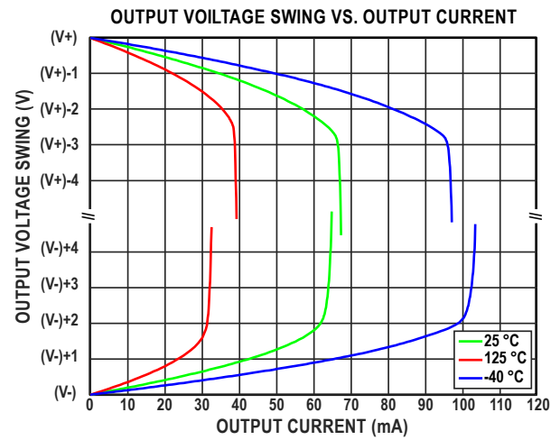
图32. 输出电压摆幅与输出电流的关系
