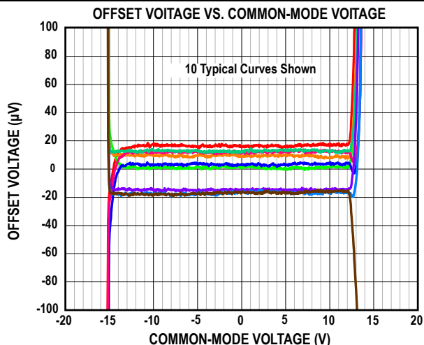
图7. 失调电压与输入共模电压的关系
