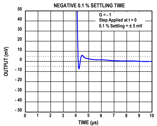
图24. 0.1%负建立时间
