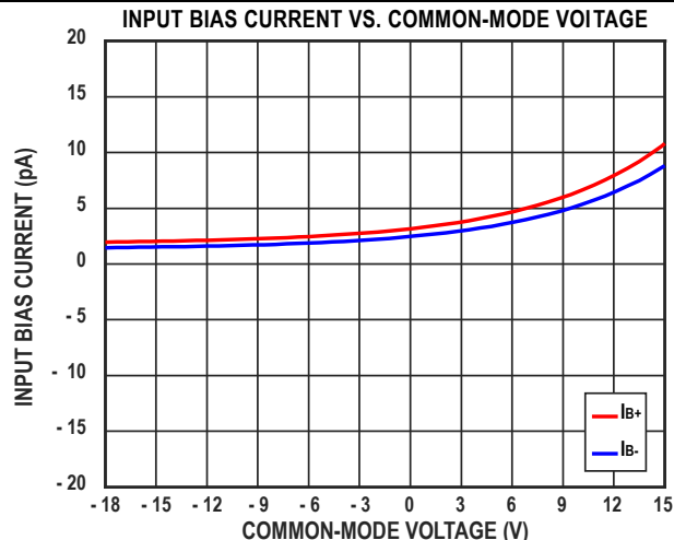
图8. 输入电流与输入共模电压的关系 ( V_{SY} = \pm 18V )
