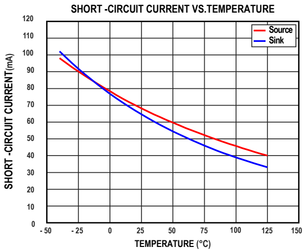
图31. 短路电流与温度的关系
