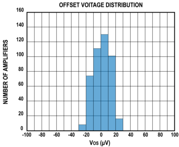
图1. 25 °C 失调电压分布，SOIC-8 封装
