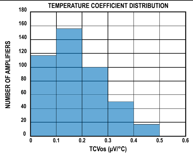
图6. 失调电压漂移分布，SOIC-8 封装
