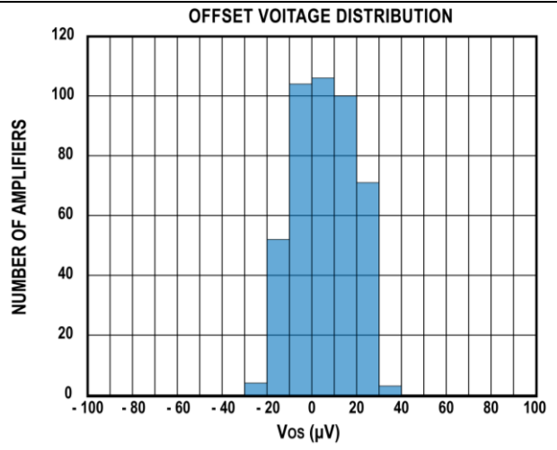
图4. 125 °C 失调电压分布，SOIC-8 封装
