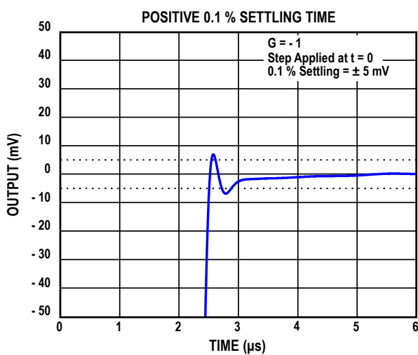
图23. 0.1%正建立时间
