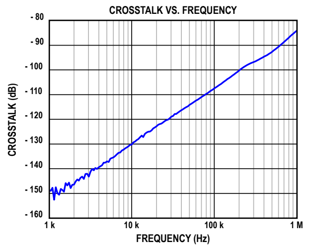
图22. 通道隔离度与频率的关系
