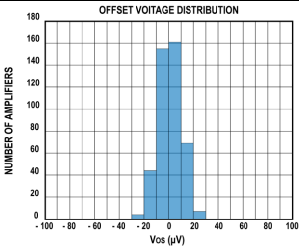
图3. 85 °C 失调电压分布，SOIC-8 封装
