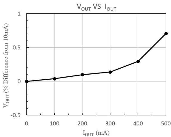
图 3 输出电压随负载电流变化 ( V_{IN}=8V )
