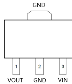
SOT89-3L(Type-B)
