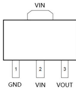
SOT89-3L(Type-A)
