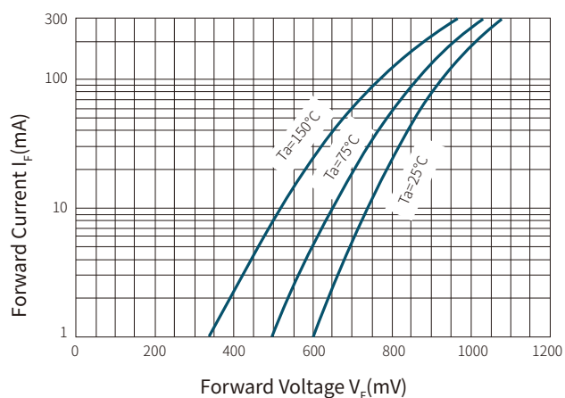
Fig.1 V_F — I_F
