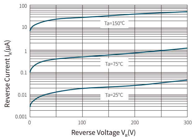
Fig.2 I_R — V_R
