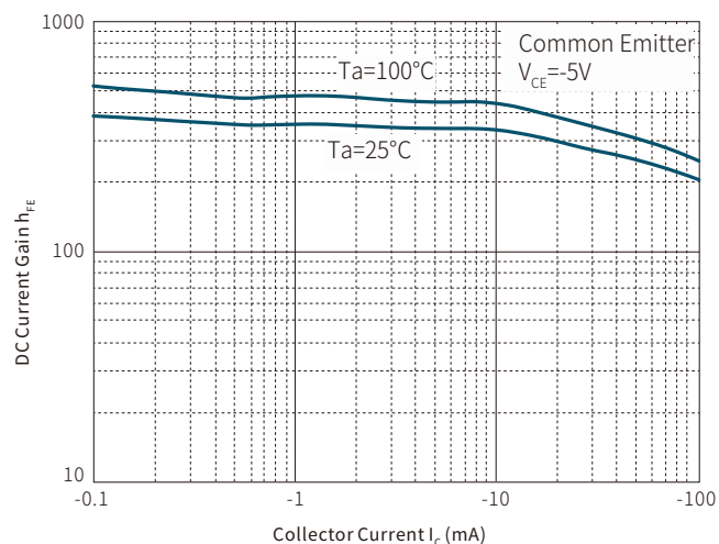
h_{FE} — I_C
