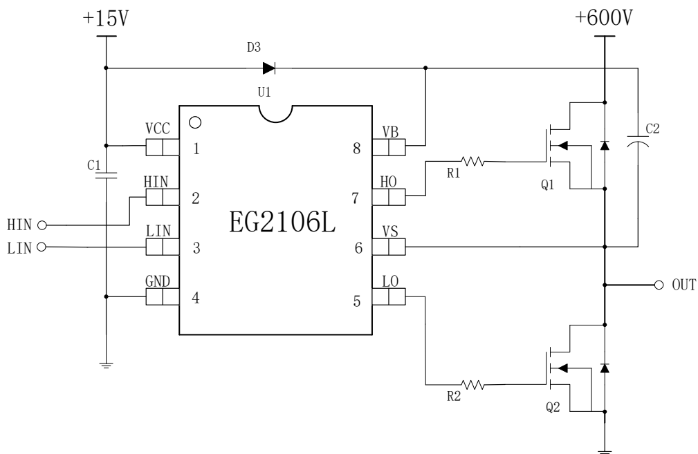
图 6-1. EG2106L 典型应用电路图
