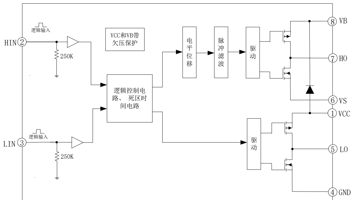
图 5-1. EG2106L 内部电路图
