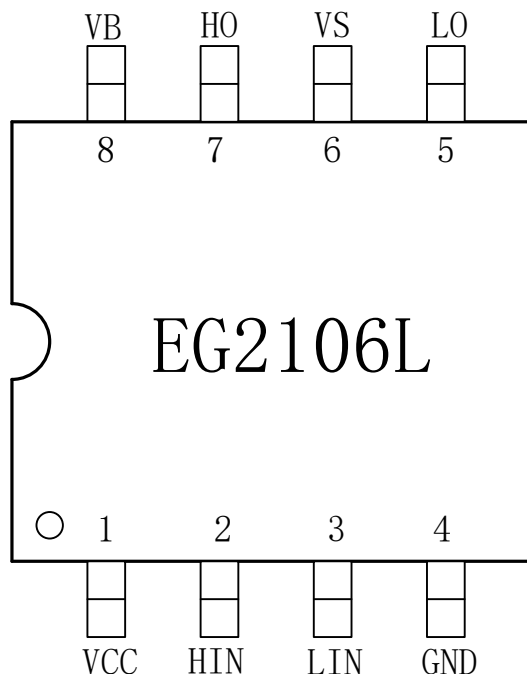
图 4-1. EG2106L 管脚定义
