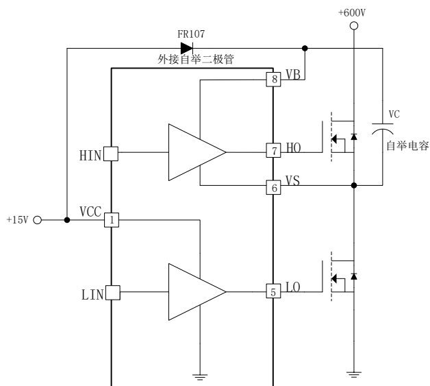
图 8-3. EG2106L 自举电路结构
