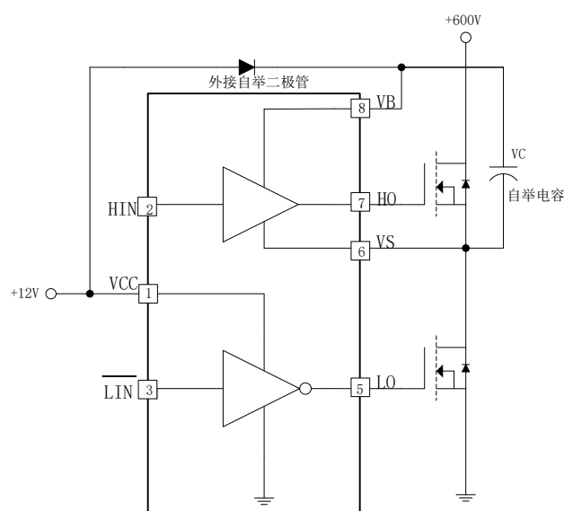
图 8-3. EG2103L 自举电路结构
