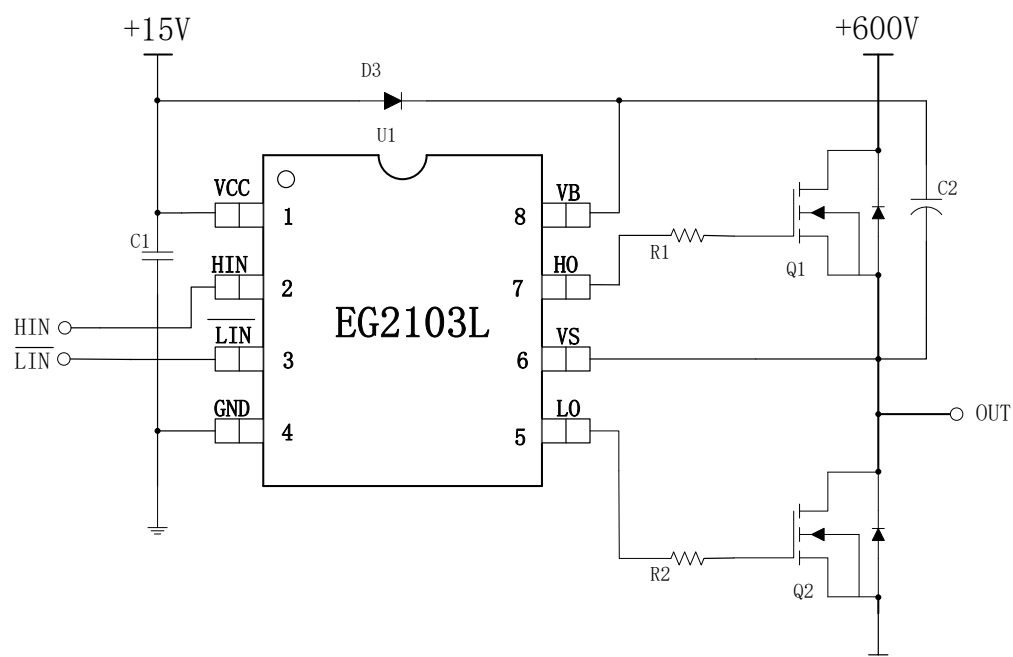
图 6-1. EG2103L 典型应用电路图
