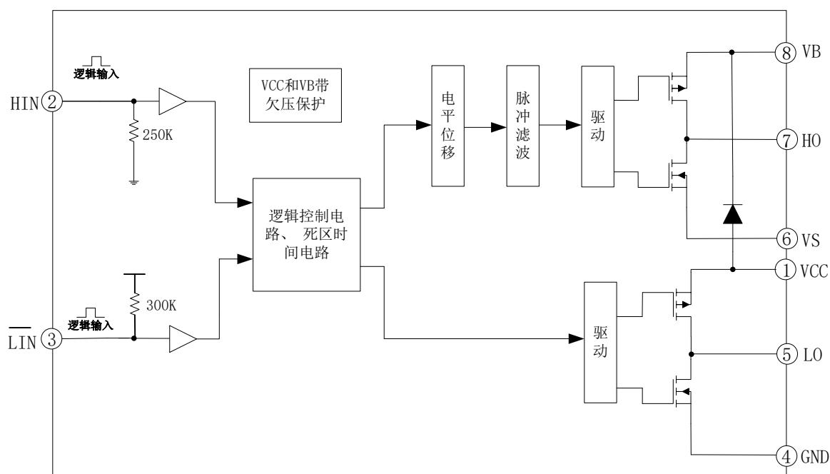
图 5-1. EG2103L 内部电路图
