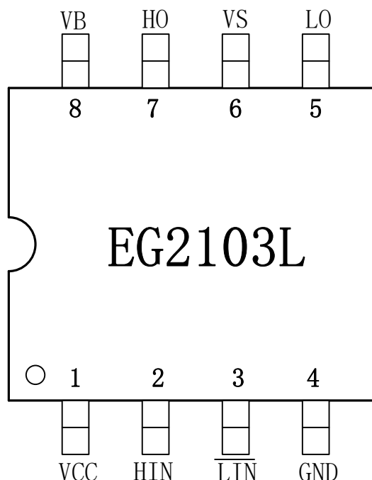
图 4-1. EG2103L 管脚定义
