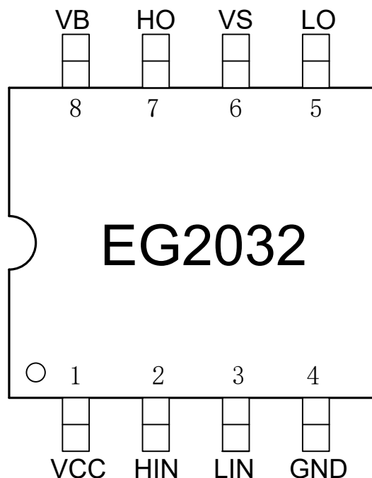
图 4-1. EG2032 管脚定义
