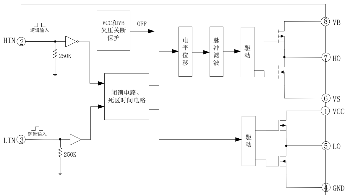
图 5-1. EG2032 内部电路图
