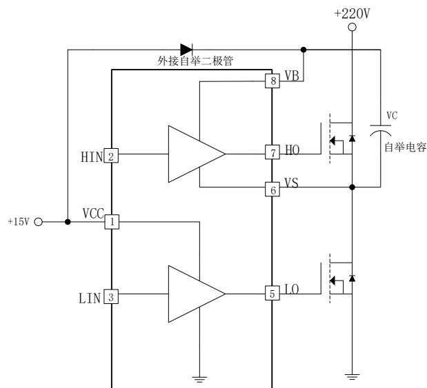
图 8-3. EG2032 自举电路结构
