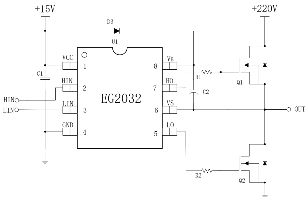
图 6-1. EG2032 典型应用电路图
