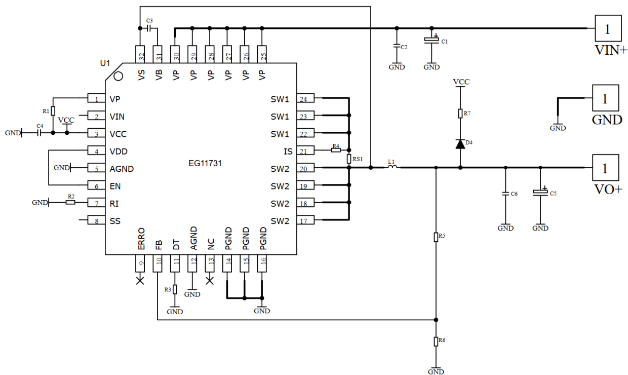
图 6-2. EG11731 外部启动电阻反馈供电典型应用图
