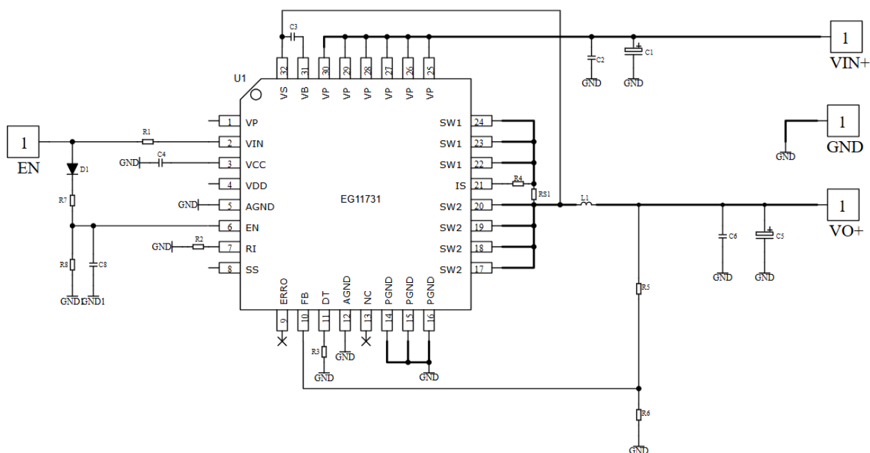
图 6-3. EG11731 关闭延时典型应用图
