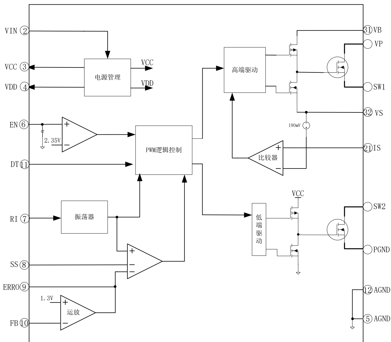
图 5-1. EG11731 内部电路图
