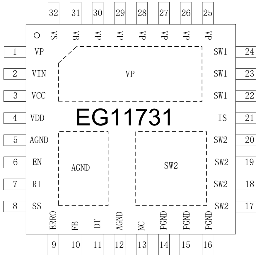
图 4-1. EG11731 管脚定义
