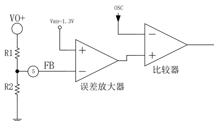
图 8.5 EG11731 输出电压调整电路
