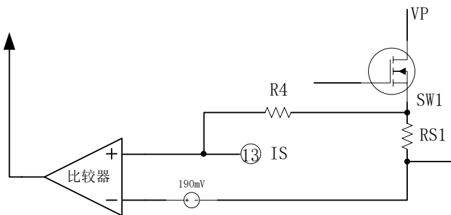
图 8.7 EG11731 峰值限流电路
