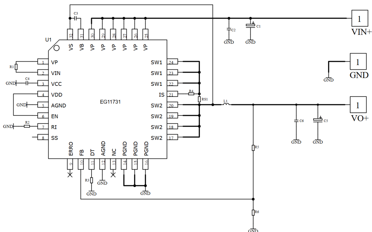
图 6-1. EG11731 VIN 快速启动供电典型应用图
