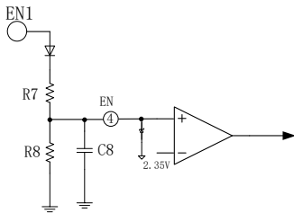
图 8.6 EG11731 关闭延时电路
