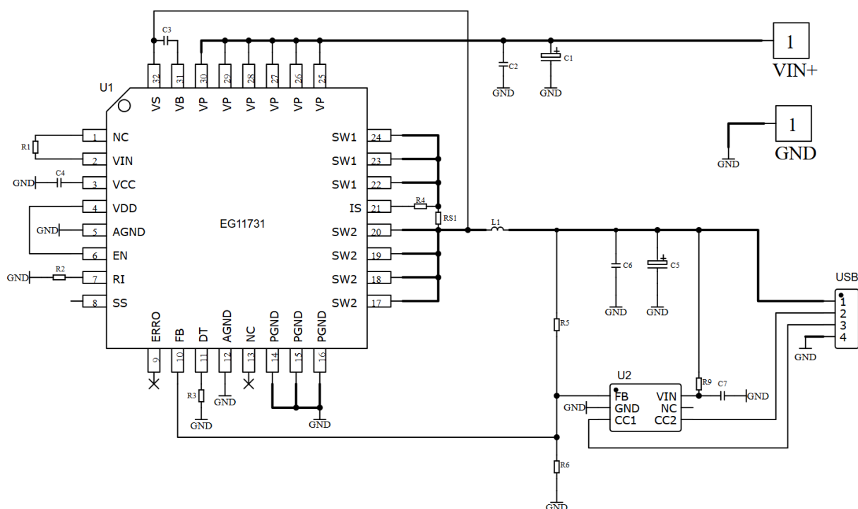
图 6-4. EG11731 快充方案典型应用图
