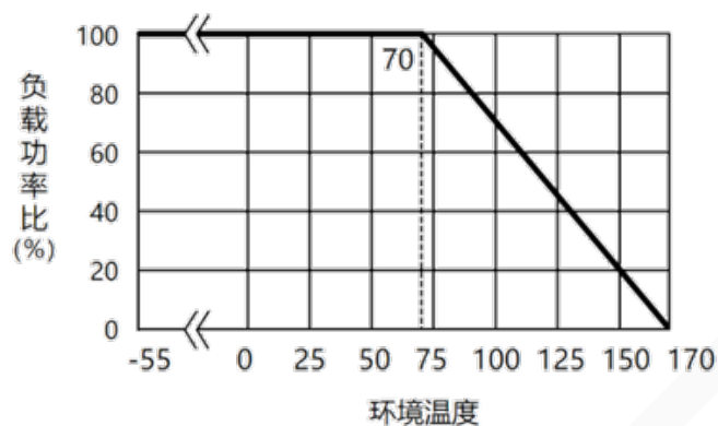
功率曲线
