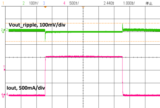
Ch2—Vout_ripple, Ch4—Iout
