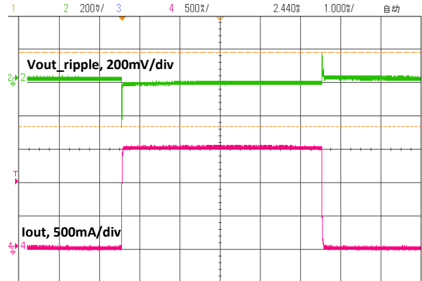
Ch2—Vout_ripple, Ch4—Iout
