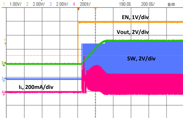
Ch1—EN, Ch2—Vout, Ch3—SW, Ch4—I L
