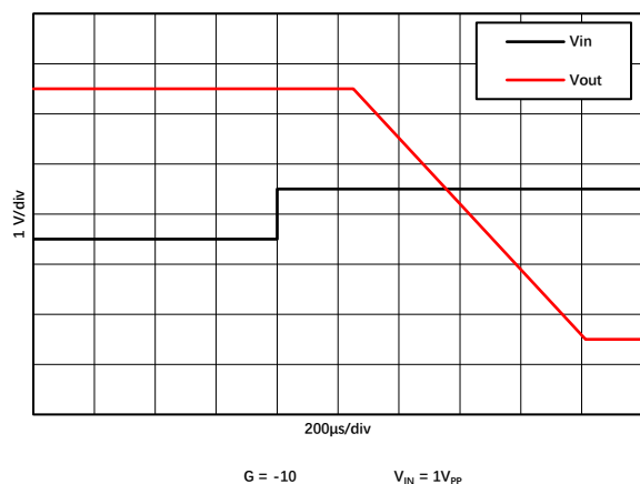
图 1.9.7. 正过载恢复
