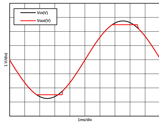
图 1.9.5. 无相位翻转
