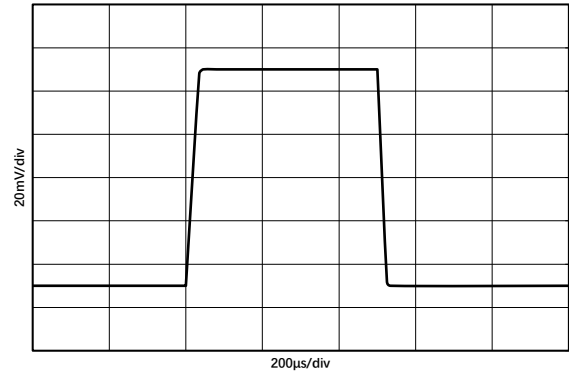
图 1.9.2. 小信号阶跃响应 @ V_S = 1.4\text{V}
