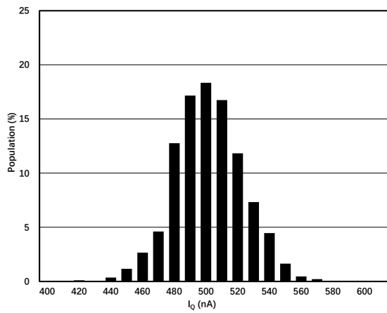
图 1.7.3. 静态电流分布图
