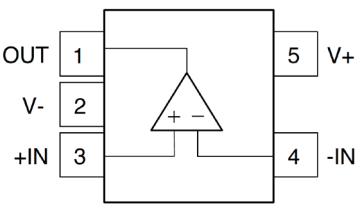
SOT23-5_A/SOT353_A
