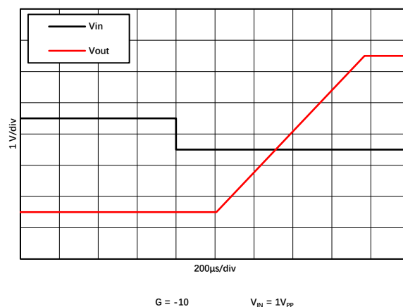
图 1.9.8. 负过载恢复
