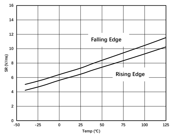
图 1.9.6. 压摆率 vs 温度
