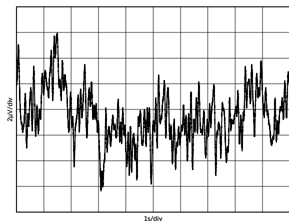
图 1.8.5. 0.1Hz 到 10Hz 噪声
