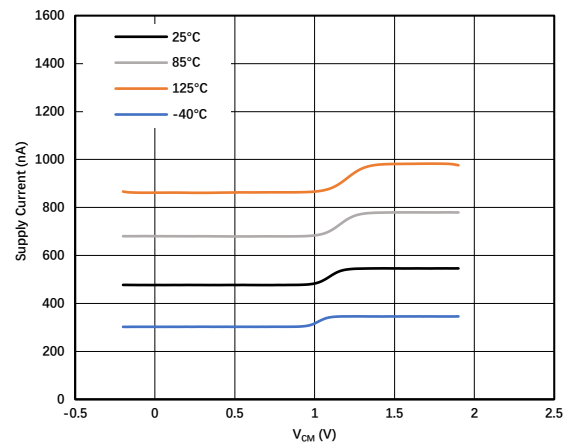
图 1.7.8. 静态电流 vs 共模电压 @ V_S = 1.6\text{V}
