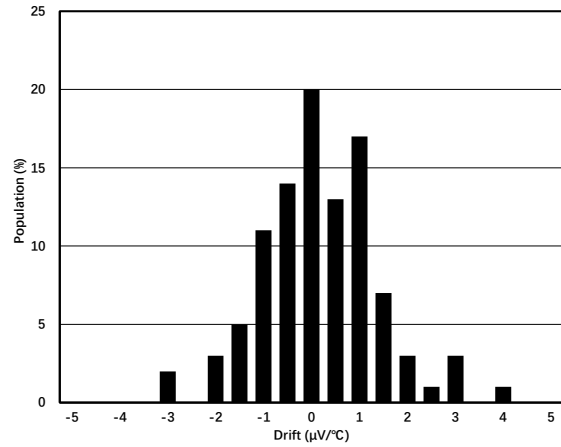
图 1.7.2. 温漂分布图
