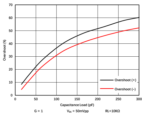
图 1.9.7. 小信号过冲与容性负载
