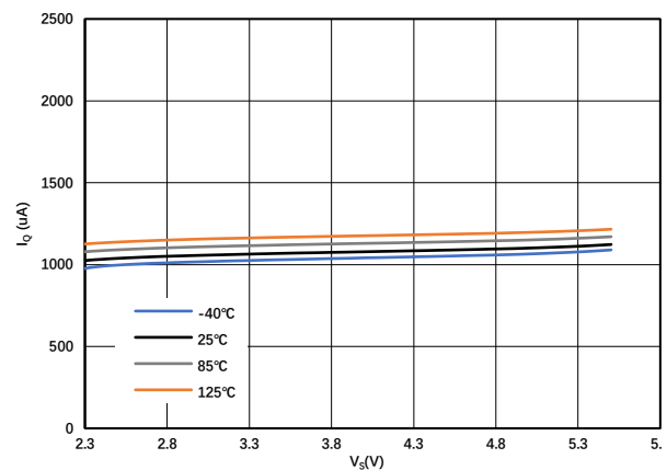
图 1.7.4. 静态电流 vs 供电电压 @ V_{CM} = 0\text{V}
