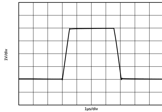
图 1.9.2. 大信号阶跃响应 @ V_S = 5\text{V}
