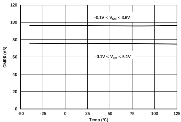
图 1.7.11. 直流 CMRR 与温度的关系 @ V_S = 5\text{V}
