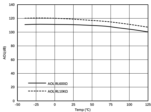
图 1.7.13. 开环增益与温度的关系 @ V_S = 5\text{V}
