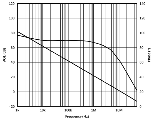
图 1.8.1. 开环增益与相位
