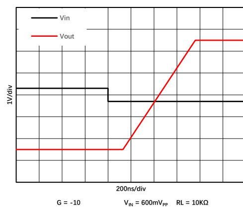
图 1.9.6. 负过载恢复
