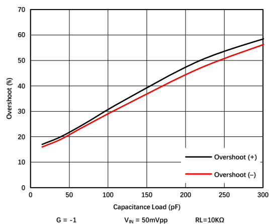
图 1.9.8. 小信号过冲与容性负载
