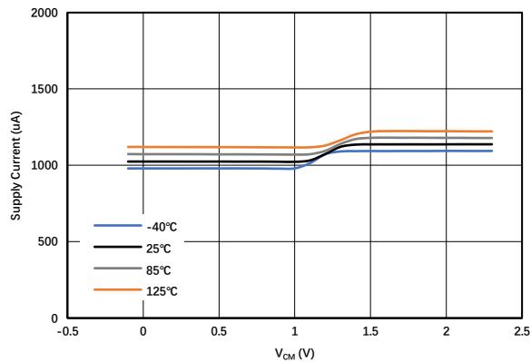
图 1.7.8. 静态电流 vs 共模电压 @ V_S = 2.3\text{V}
