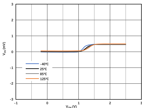
图 1.7.10. 输入失调电压 vs 共模电压 @ V_S = 2.3\text{V}
