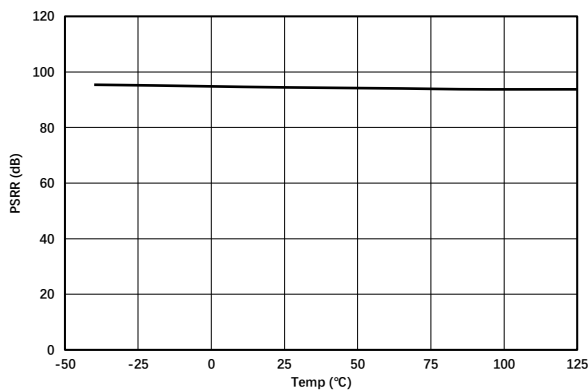
图 1.7.12. 直流 PSRR 与温度的关系 @ V_S = 2.3\text{V} 到 5.5\text{V}
