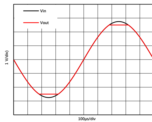
图 1.9.4. 无相位翻转
