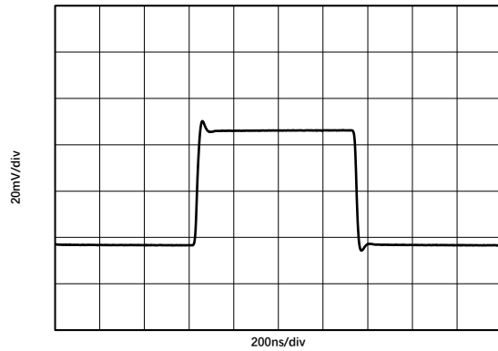
图 1.9.1. 小信号阶跃响应 @ V_S = 5\text{V}
