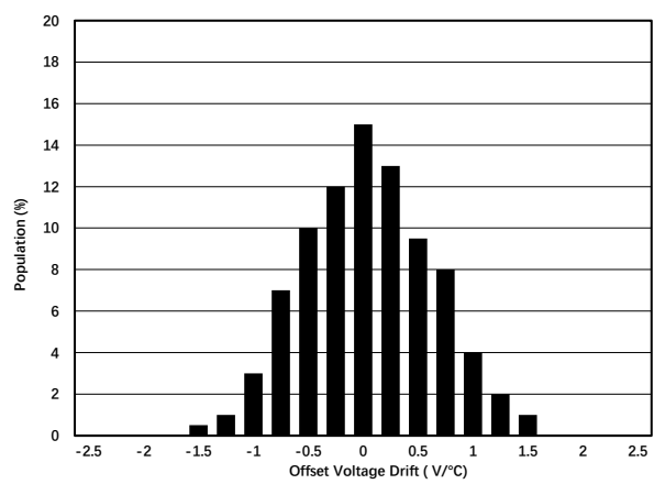
图 1.7.2. 温漂分布图
