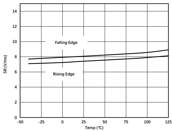
图 1.9.3. 压摆率 vs 温度
