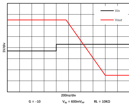
图 1.9.5. 正过载恢复
