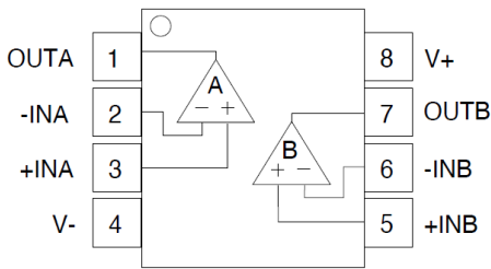
SOP8/MSOP8
