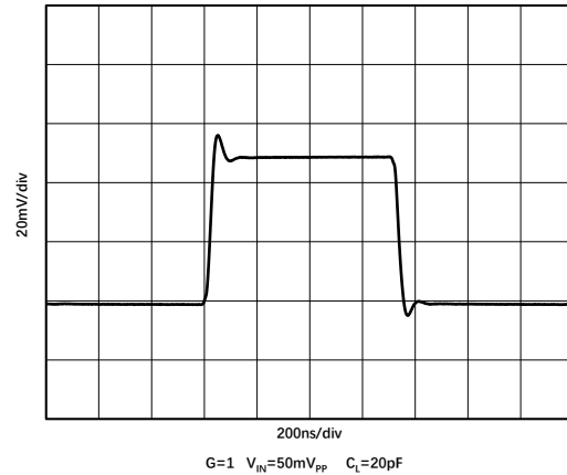
图 1.9.2. 小信号阶跃响应 @ V_S = 1.7\text{V}
