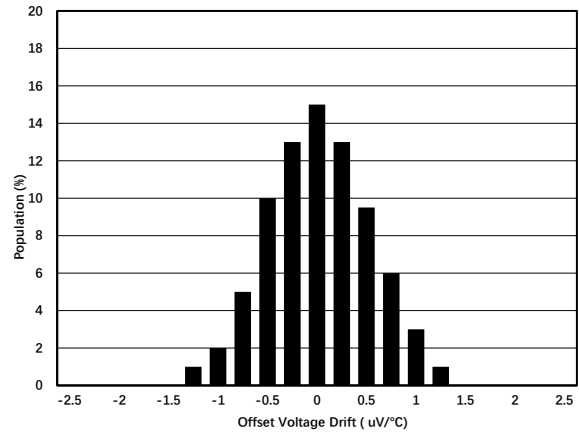
图 1.7.2. 温漂分布图
