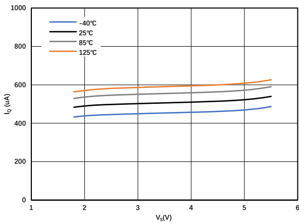
图 1.7.4. 静态电流 vs 供电电压 @ V_{CM} = 0\text{V}
