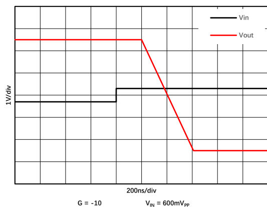
图 1.9.7. 正过载恢复
