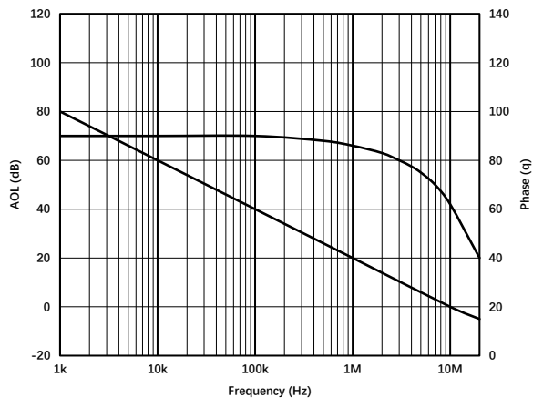
图 1.8.1. 开环增益与相位
