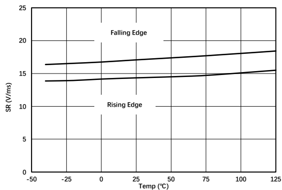
图 1.9.5. 压摆率 vs 温度
