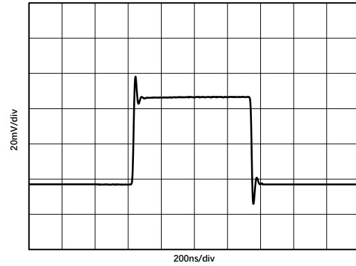
G=1 V_{IN}=50\text{mV}_{PP} C_L=20\text{pF} R_L=10\text{K}\Omega 图 1.9.2. 小信号阶跃响应 @ V_S = 2.5\text{V}
