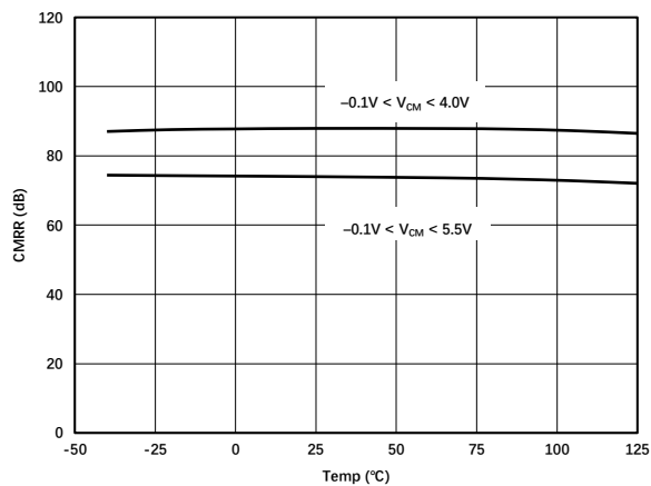
图 1.7.11. 直流 CMRR 与温度的关系 @ V_S = 5.5\text{V}
