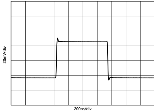
G=1 V_{IN}=50\text{mV}_{PP} C_L=20\text{pF} R_L=10\text{K}\Omega 图 1.9.1. 小信号阶跃响应 @ V_S = 5\text{V}
