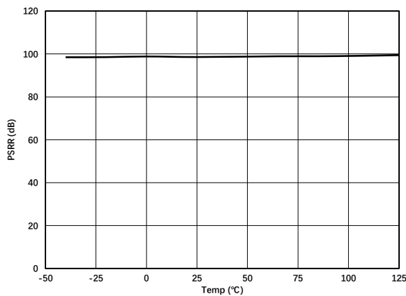
图 1.7.12. 直流 PSRR 与温度的关系 @ V_S = 2.5\text{V} 到 5.5\text{V}
