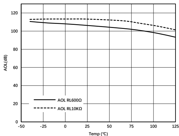
图 1.7.13. 开环增益与温度的关系 @ V_S = 5\text{V}
