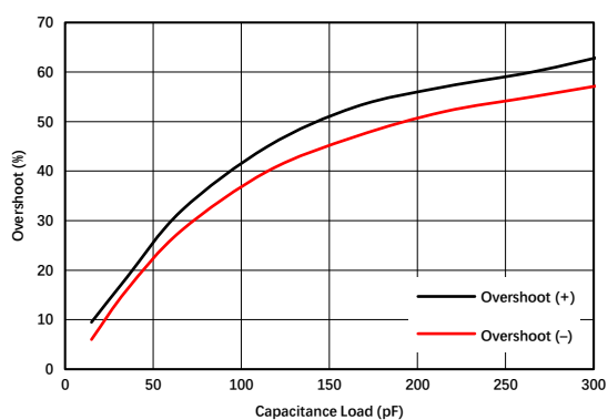
图 1.9.8. 小信号过冲与容性负载
