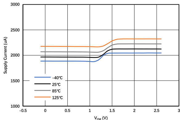
图 1.7.8. 静态电流 vs 共模电压 @ V_S = 2.5\text{V}
