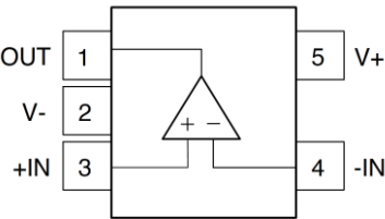
SOT23-5_A/SOT353_A
