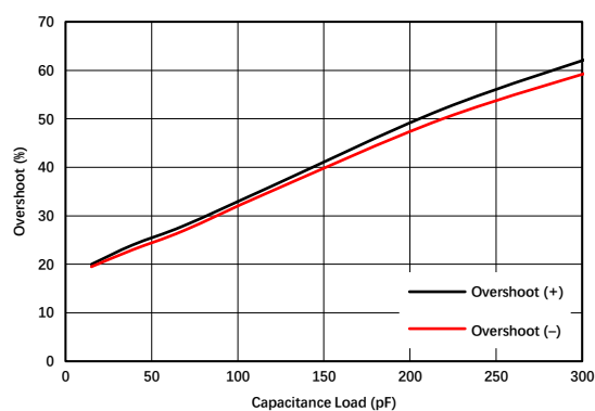
图 1.9.9. 小信号过冲与容性负载
