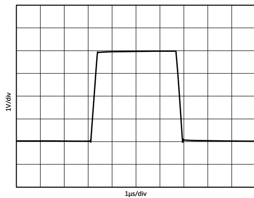
G=1 V_{IN}=4\text{V}_{PP} C_L=20\text{pF} R_L=10\text{K}\Omega 图 1.9.3. 大信号阶跃响应 @ V_S = 5\text{V}
