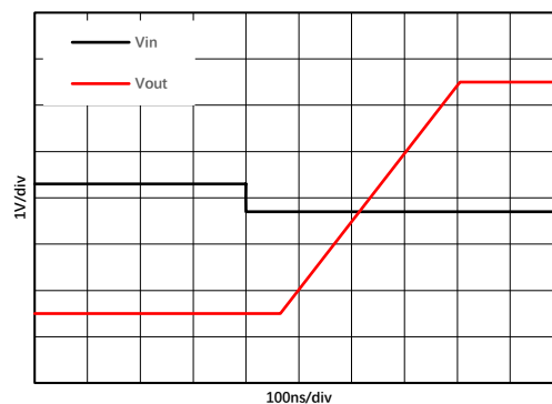
图 1.9.7. 负过载恢复
