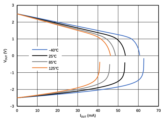
图 1.7.15. 输出电压 vs 输出电流 @ V_S = 5\text{V}
