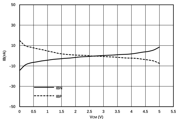
图 1.7.5. 输入偏置电流 vs 共模电压 @ V_S = 5\text{V}
