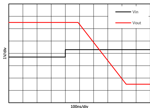
图 1.9.6. 正过载恢复
