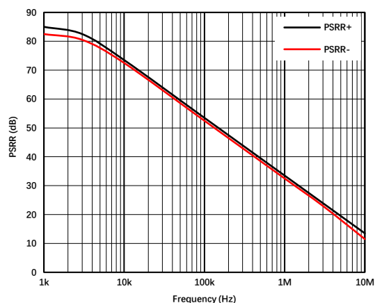
图 1.8.2. PSRR vs 频率
