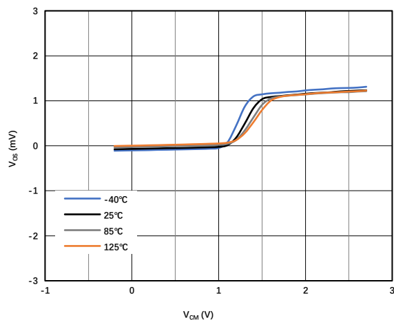
图 1.7.10. 输入失调电压 vs 共模电压 @ V_S = 2.5\text{V}
