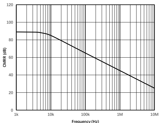
图 1.8.3. CMRR vs 频率
