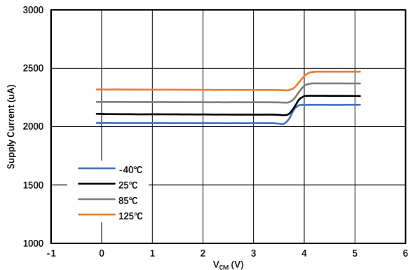
图 1.7.7. 静态电流 vs 共模电压 @ V_S = 5\text{V}
