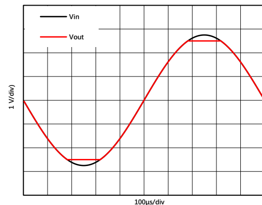
图 1.9.4. 无相位翻转
