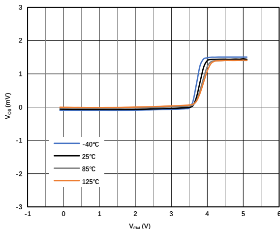
图 1.7.9. 输入失调电压 vs 共模电压 @ V_S = 5\text{V}
