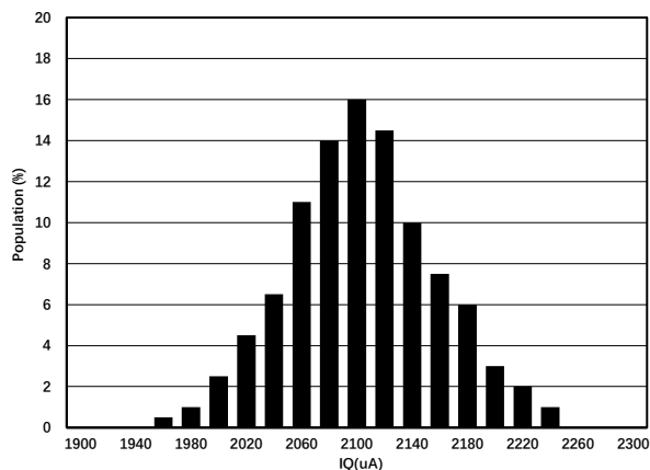
图 1.7.3. 静态电流分布图
