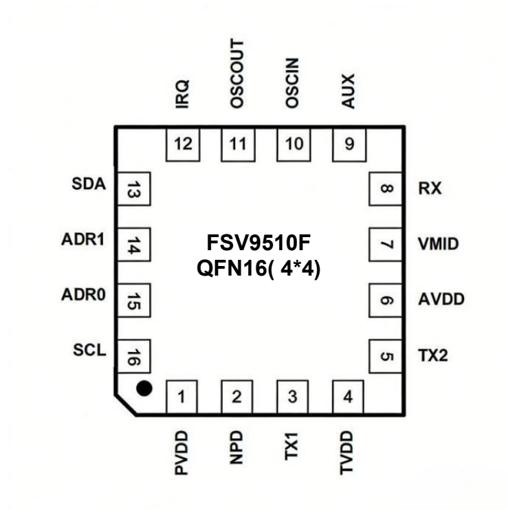
◆ 图 1 QFN16 封装管脚
