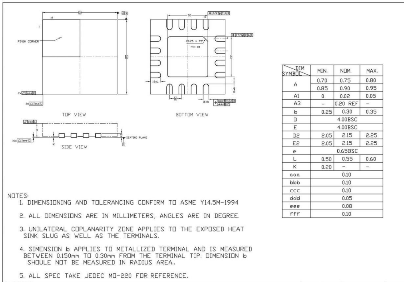
◆ 图 2 QFN16 封装尺寸图
