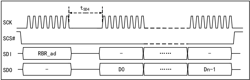
图 9-5 SPI 模式读 FIFO
