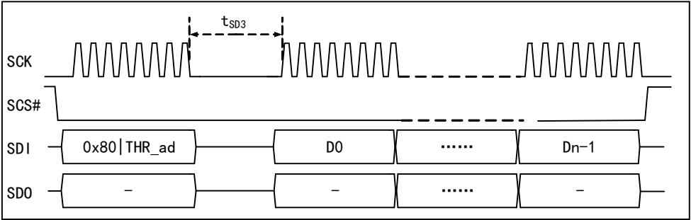
图 9-4 SPI 模式写 FIFO
