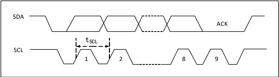
图 9-1 IIC 模式时序
