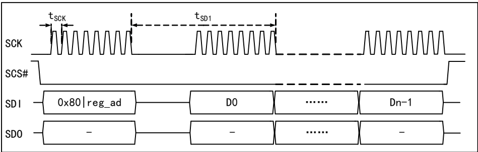
图 9-2 SPI 模式写寄存器
