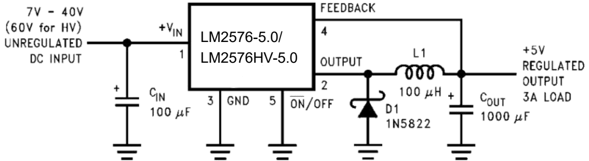
图 1、典型应用
