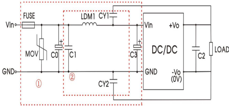
图 1 EMC 推荐电路
