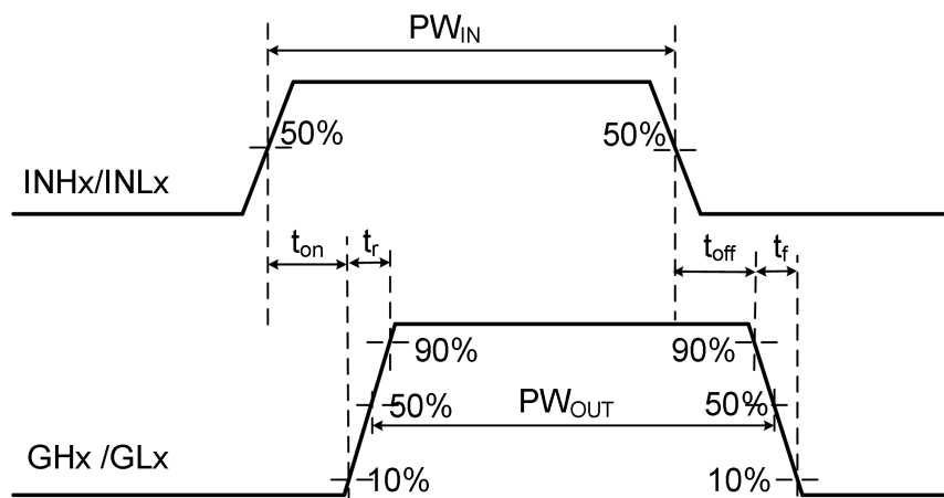
图 8-3 传输延时波形定义
