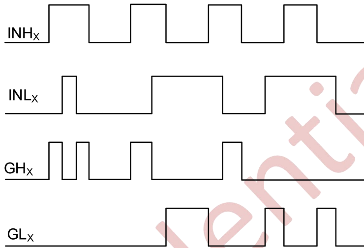
图 8-1 同向输入输出时序波形
