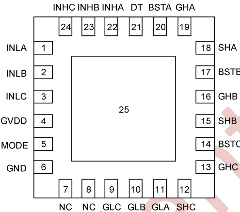
图 6-1 24 脚 QFN24 顶视图
