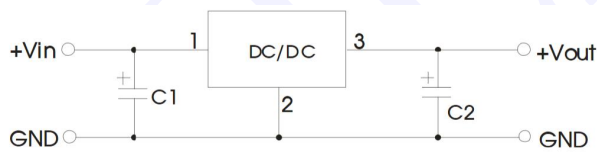
正输出应用电路
