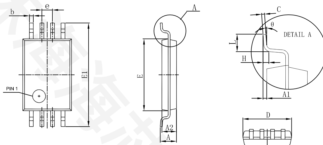
TSSOP-8
