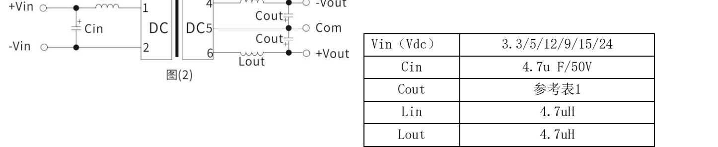
推荐 EMI 参考电路值详（表 2）
