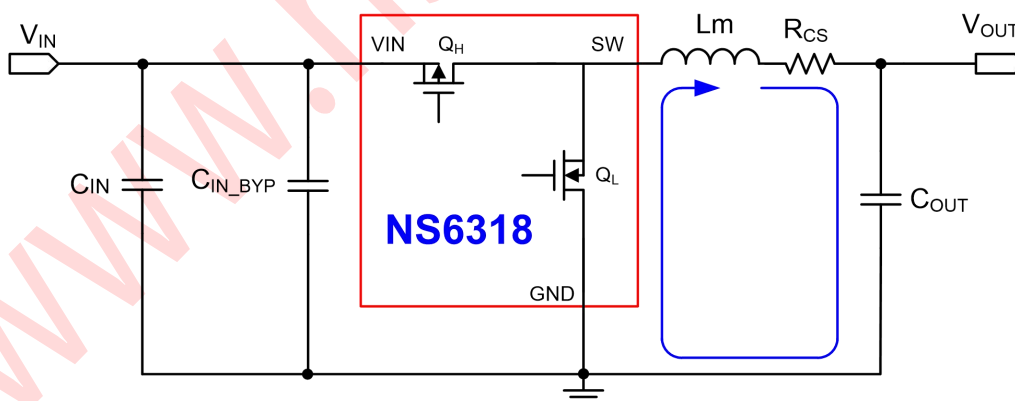
NMOS管 Q_L 导通时电感储能释放路径
