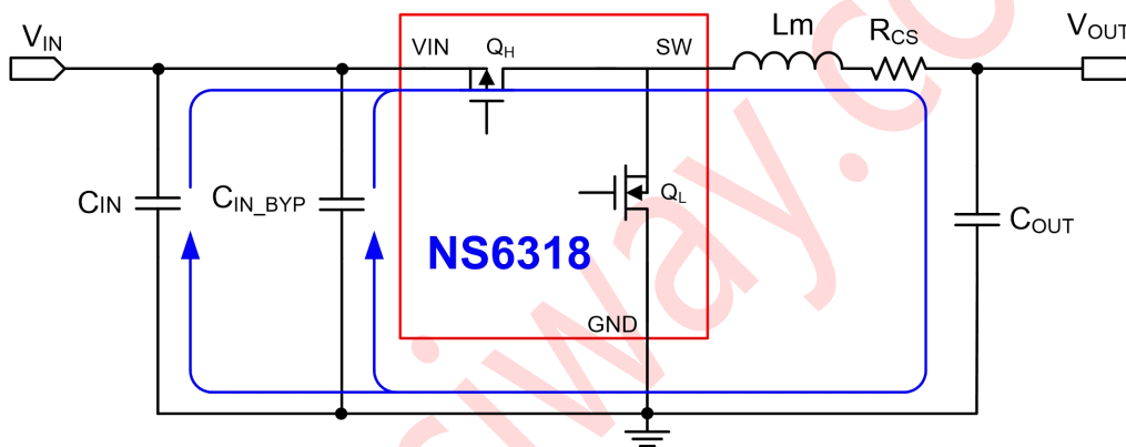
PMOS管 Q_H 导通时电感储能路径
